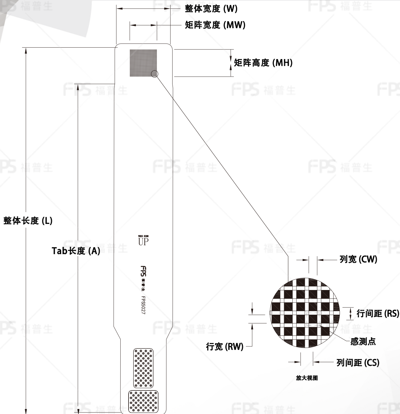
外形尺寸
