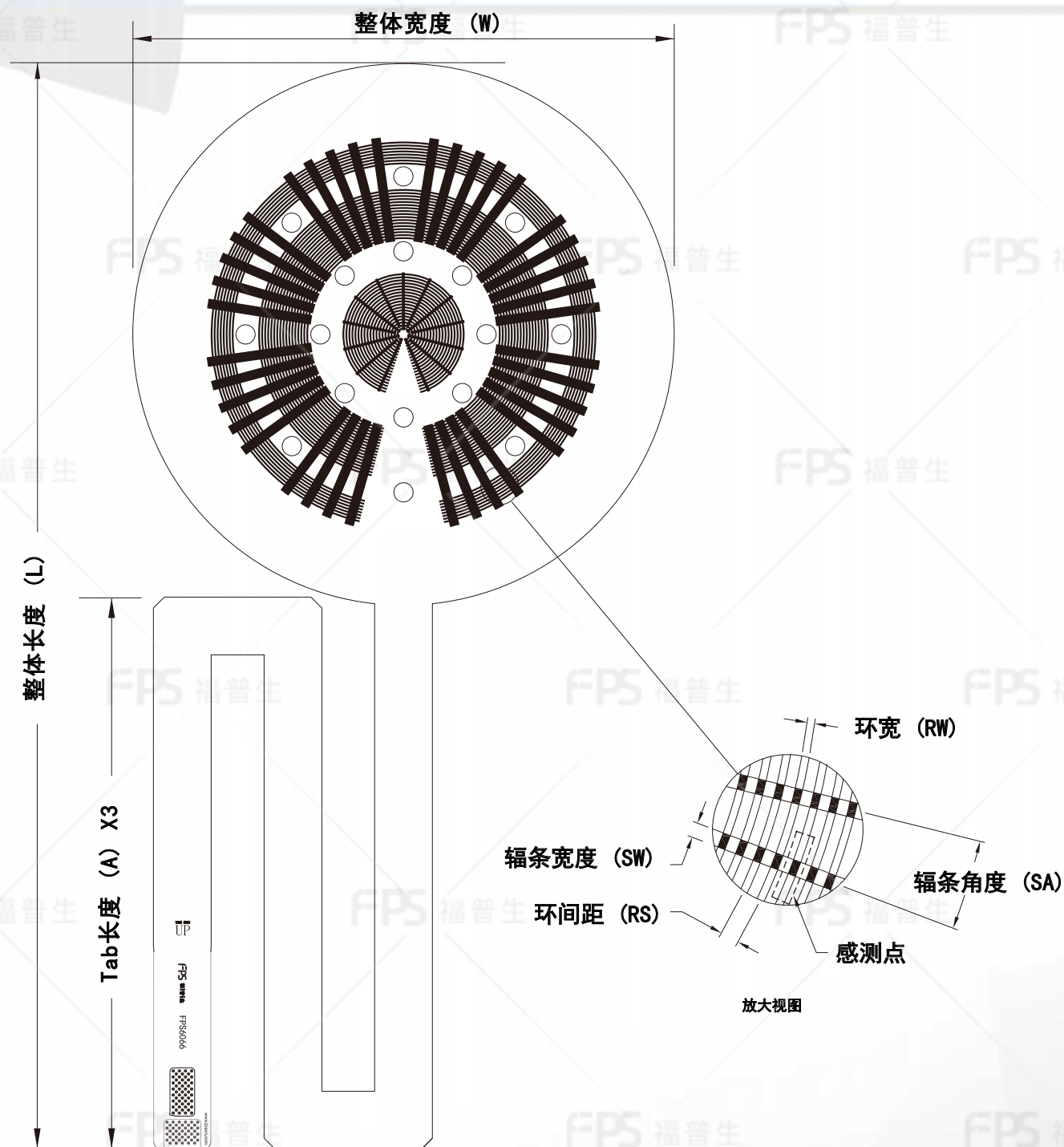
外形尺寸
