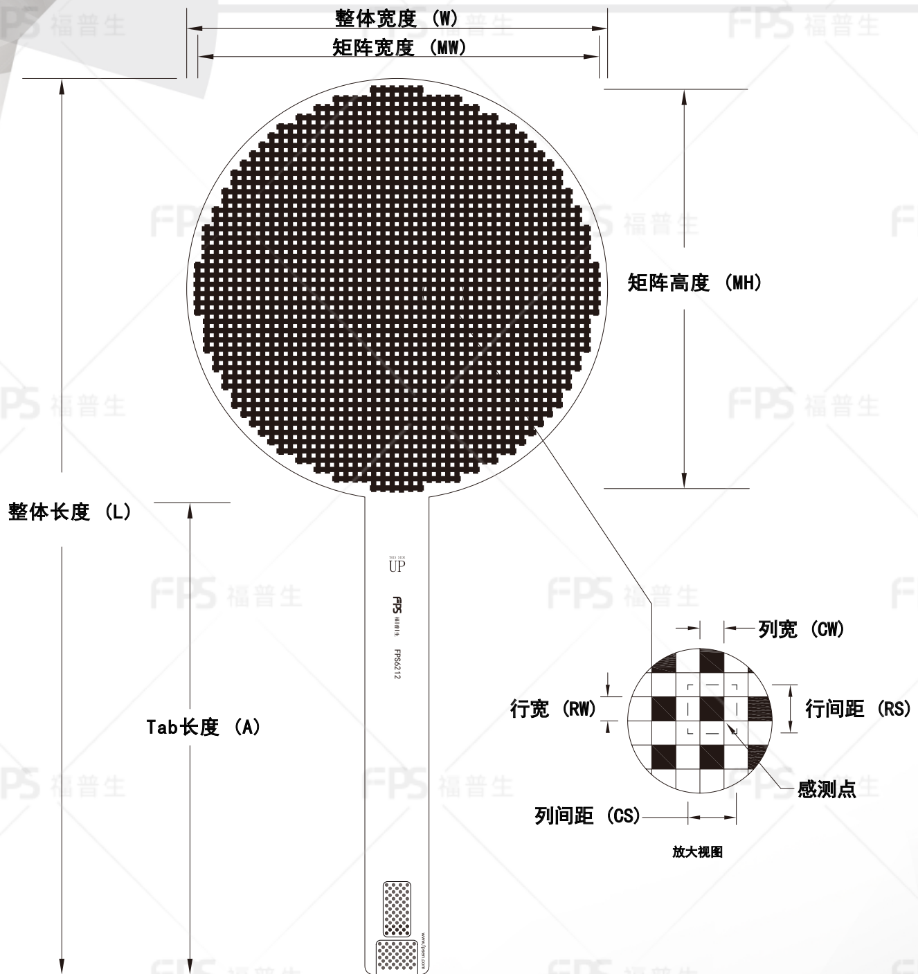
外形尺寸
