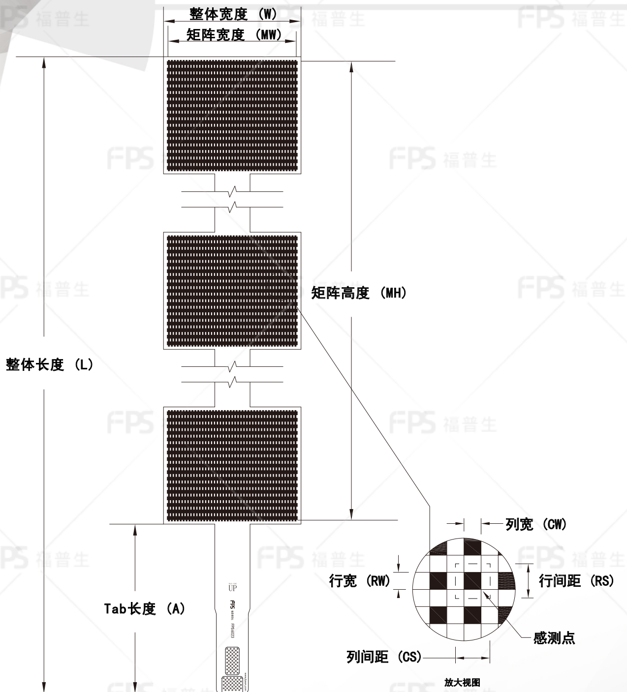
外形尺寸
