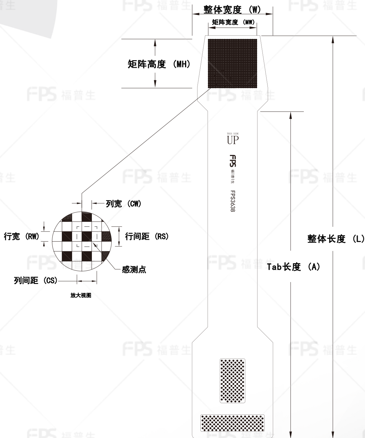
外形尺寸
