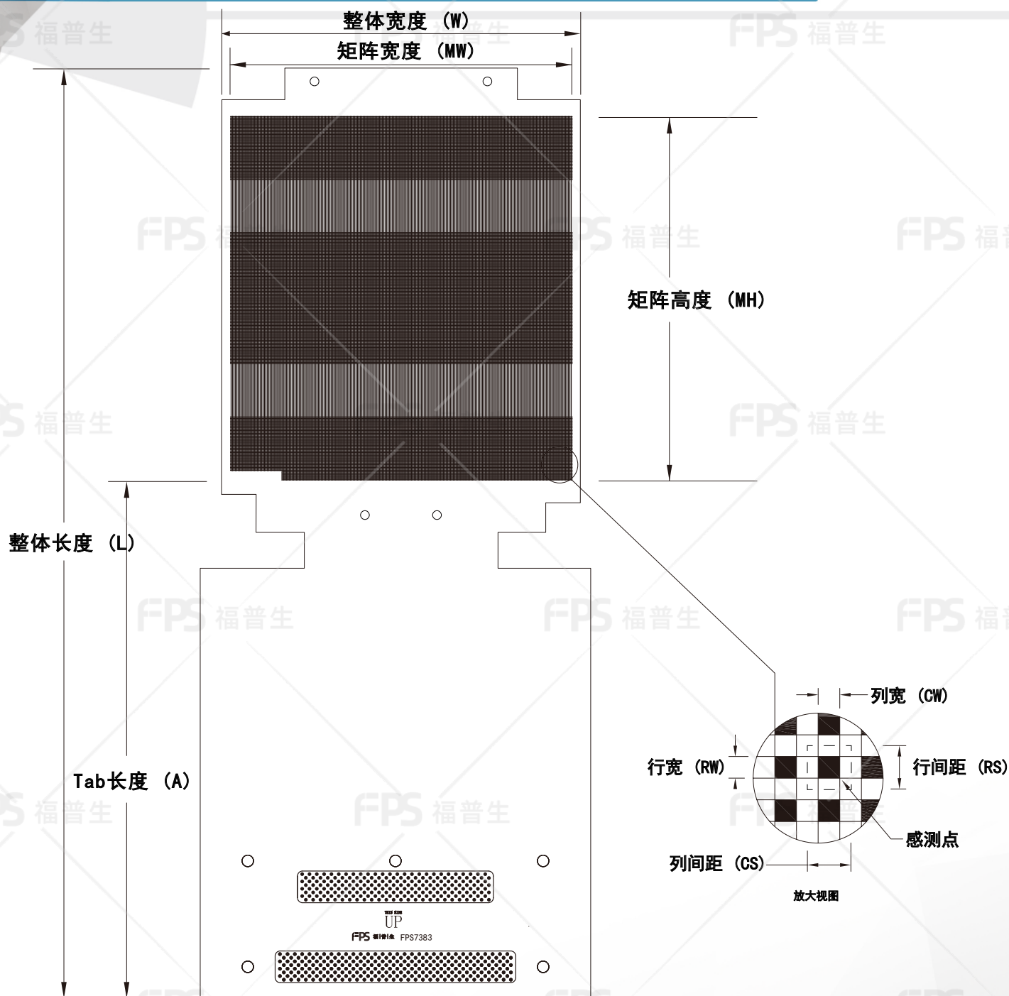
外形尺寸
