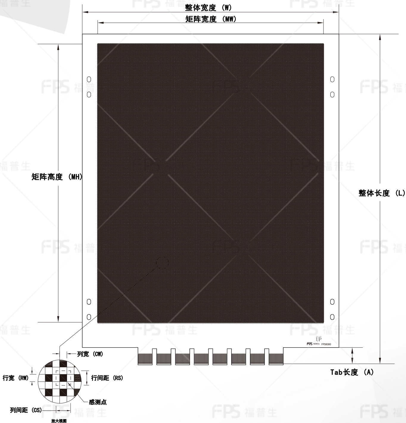
外形尺寸
