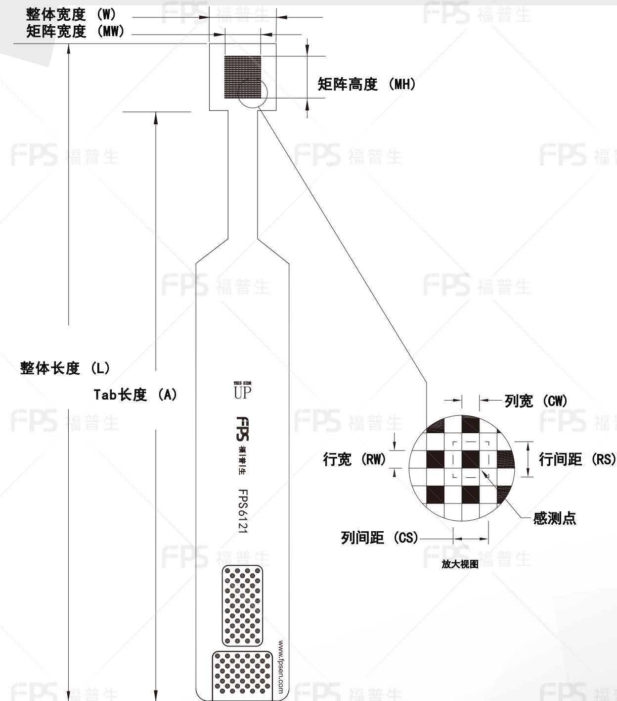
传感区参数
