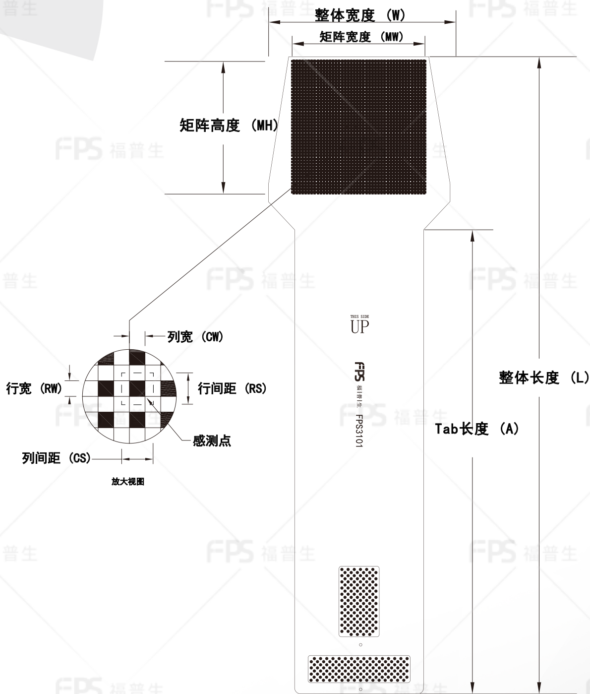
外形尺寸
