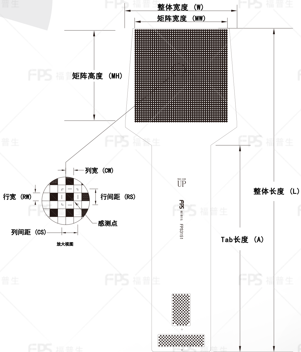
外形尺寸
