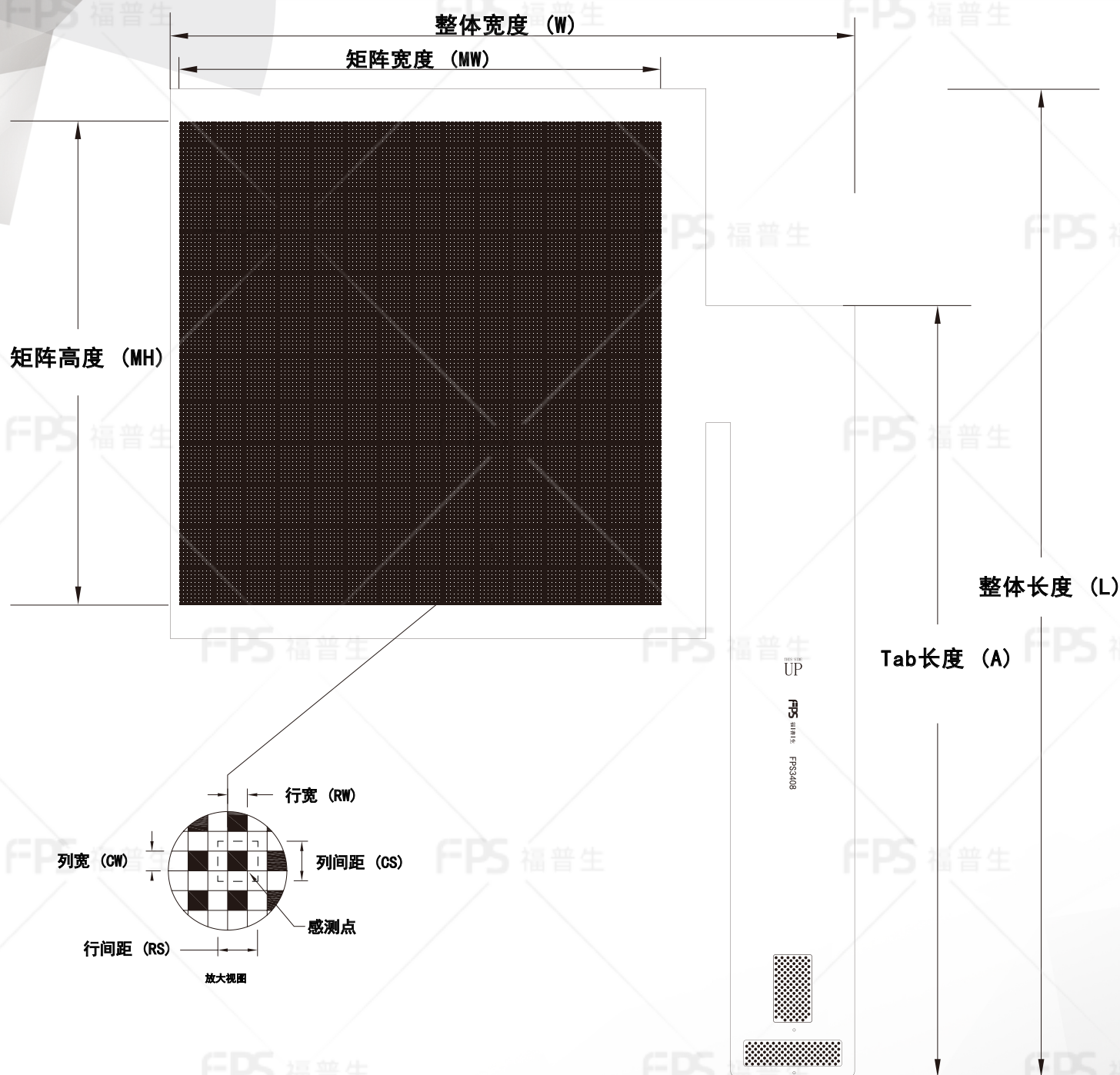
外形尺寸
