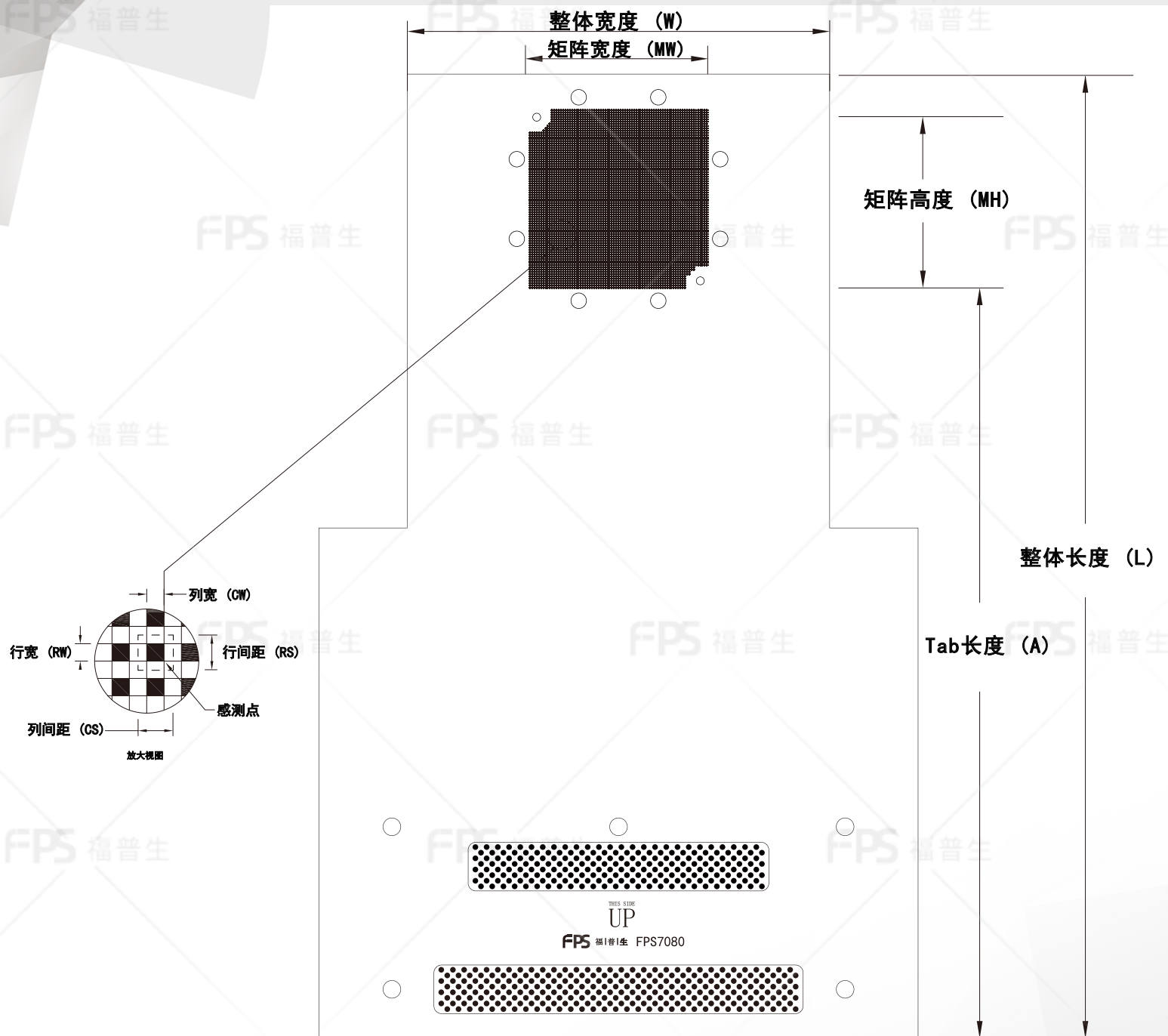
外形尺寸
