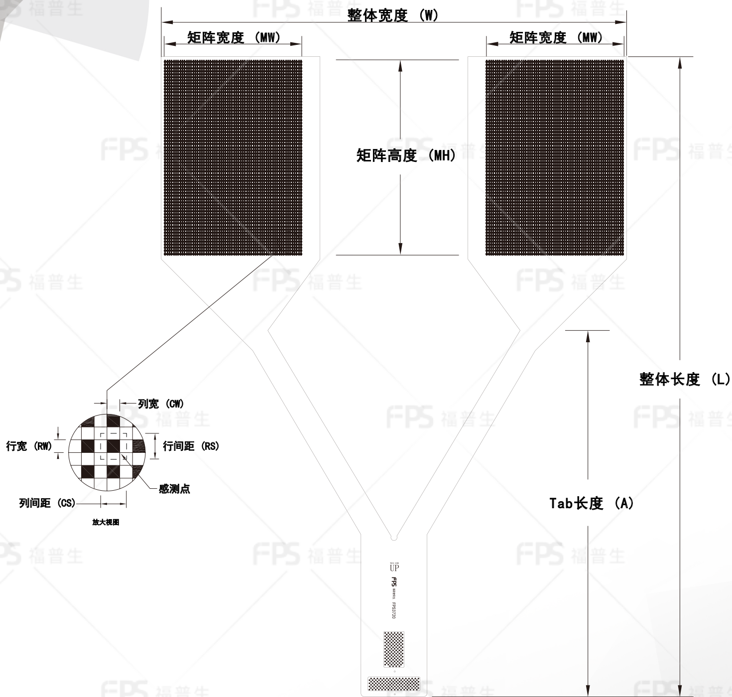
外形尺寸
