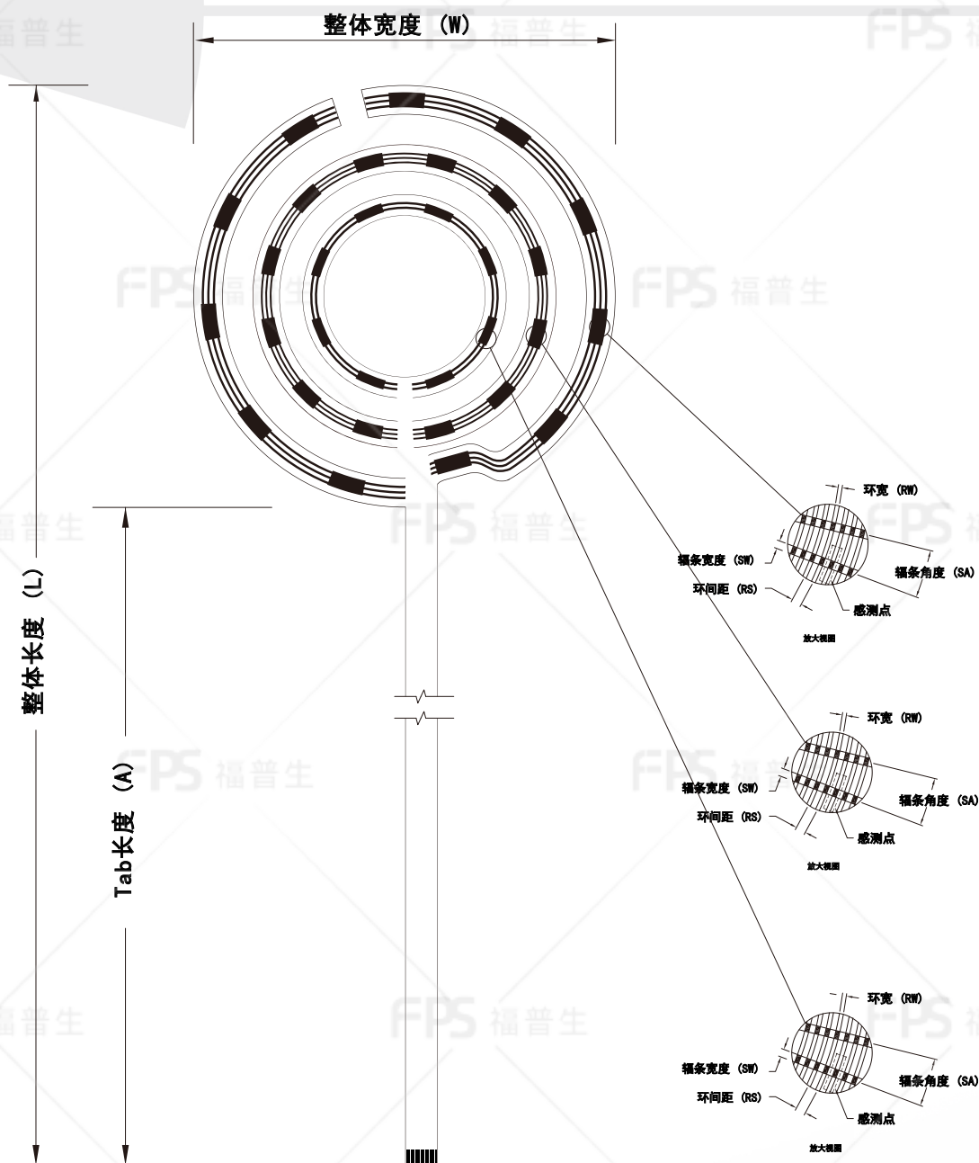
外形尺寸
