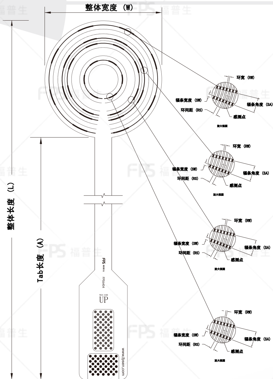
外形尺寸
