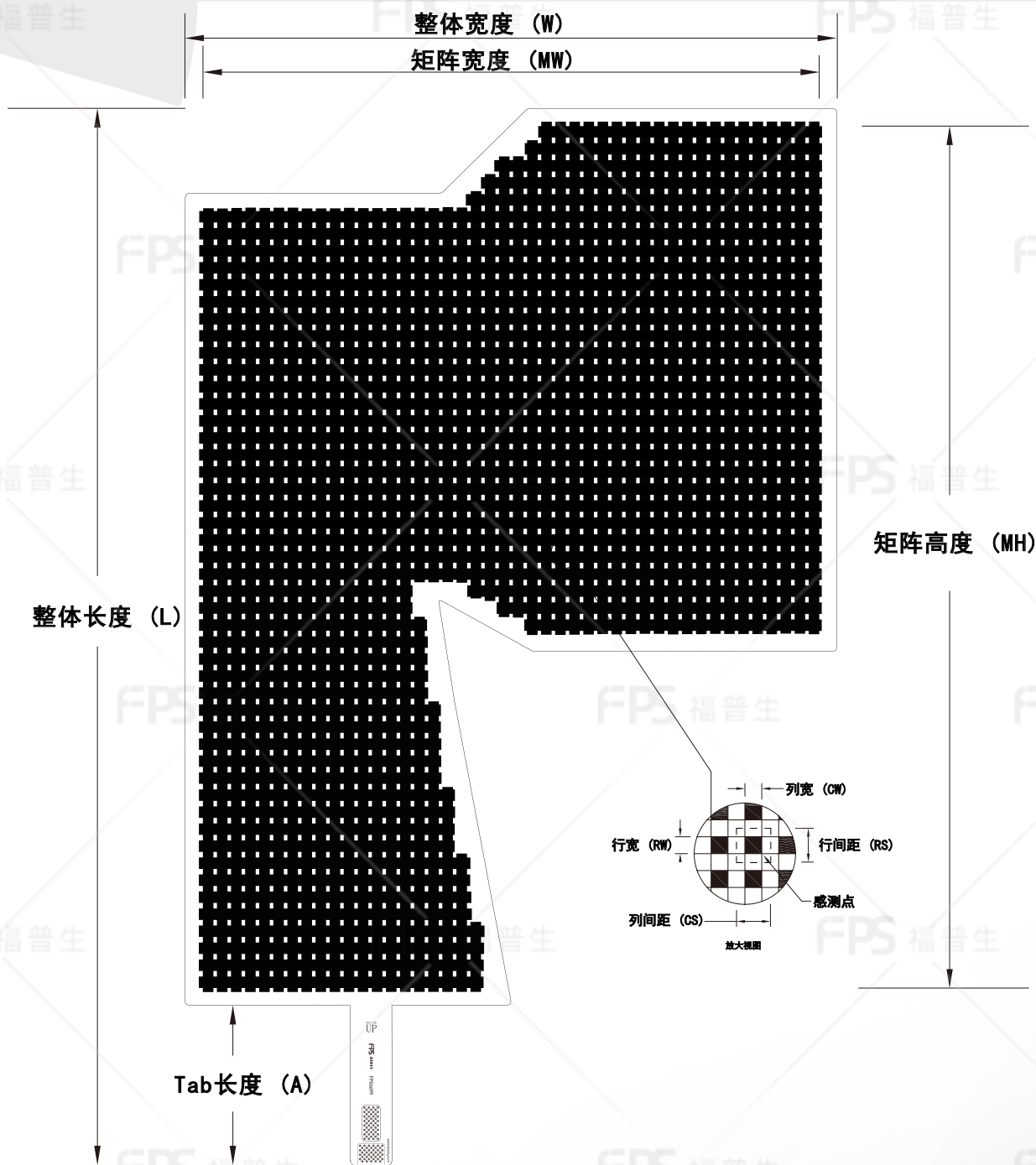
外形尺寸
