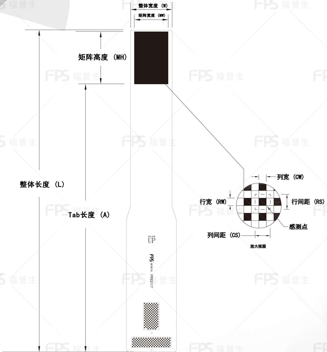
外形尺寸
