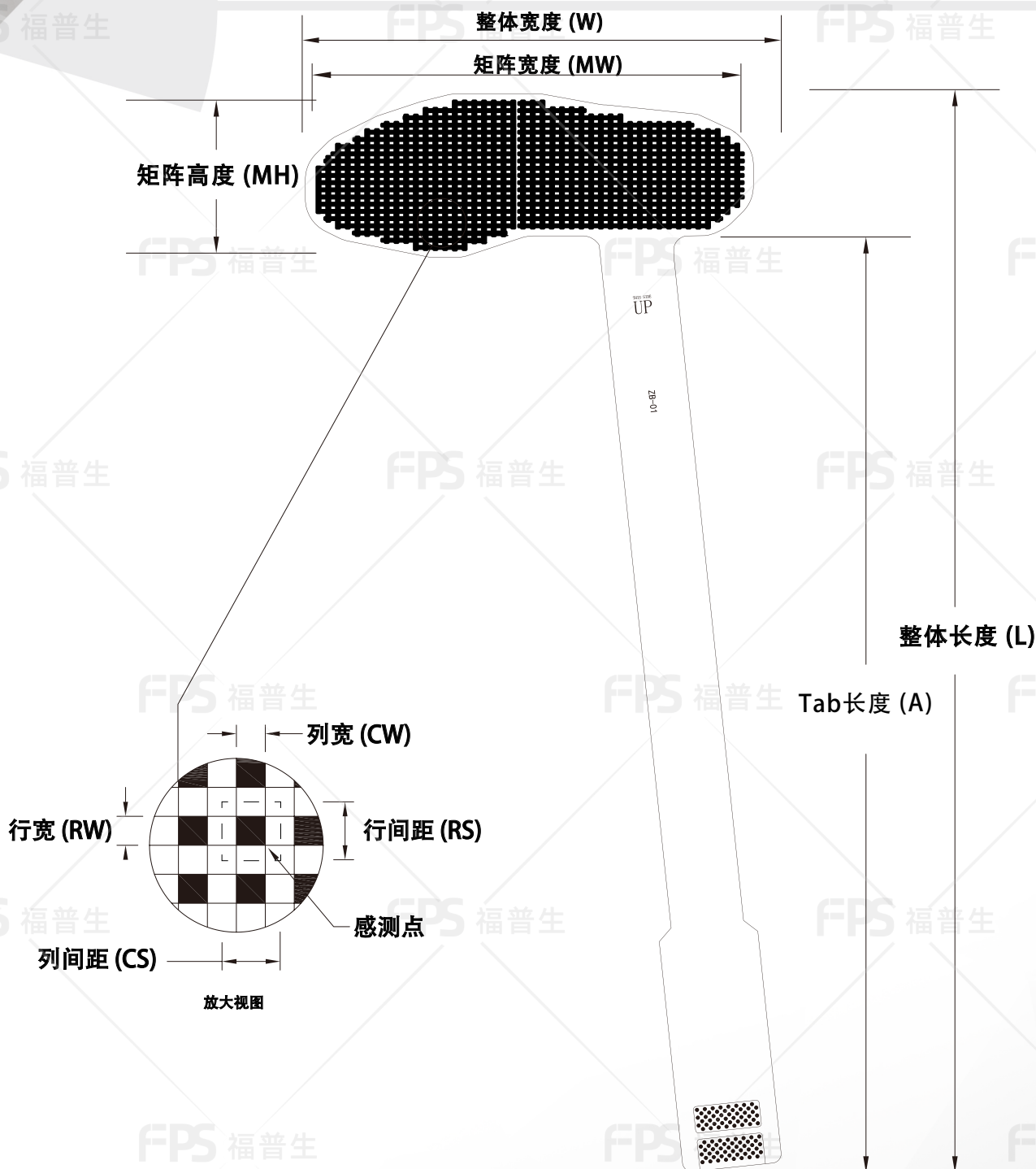
外形尺寸
