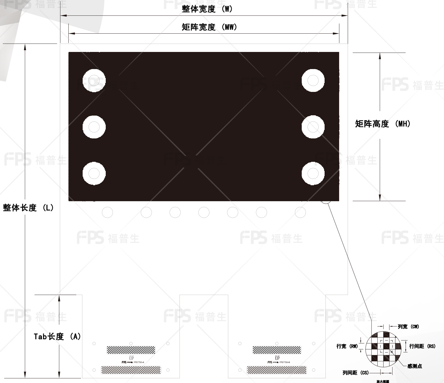
外形尺寸
