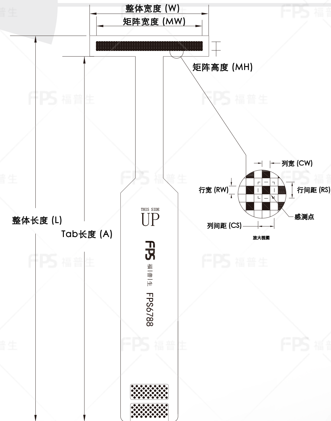
外形尺寸
