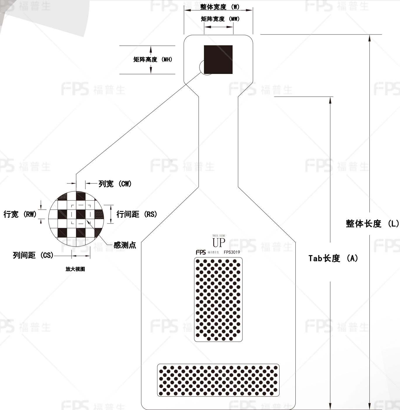
外形尺寸
