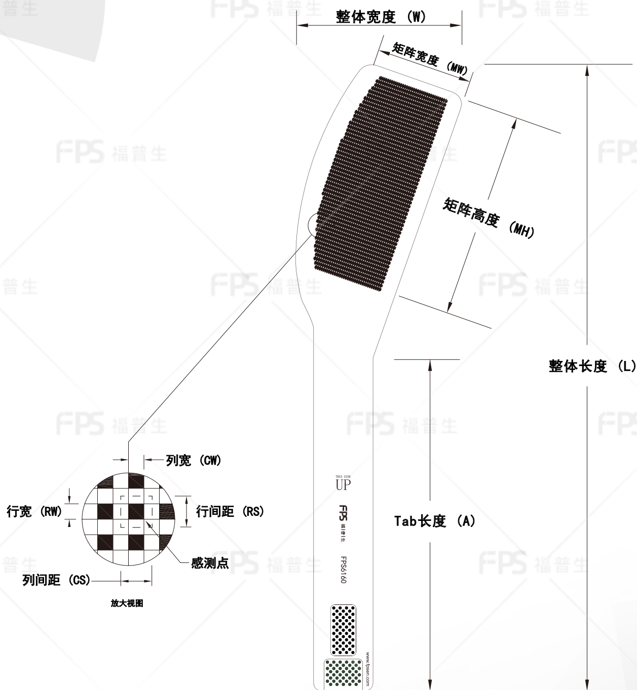
外形尺寸
