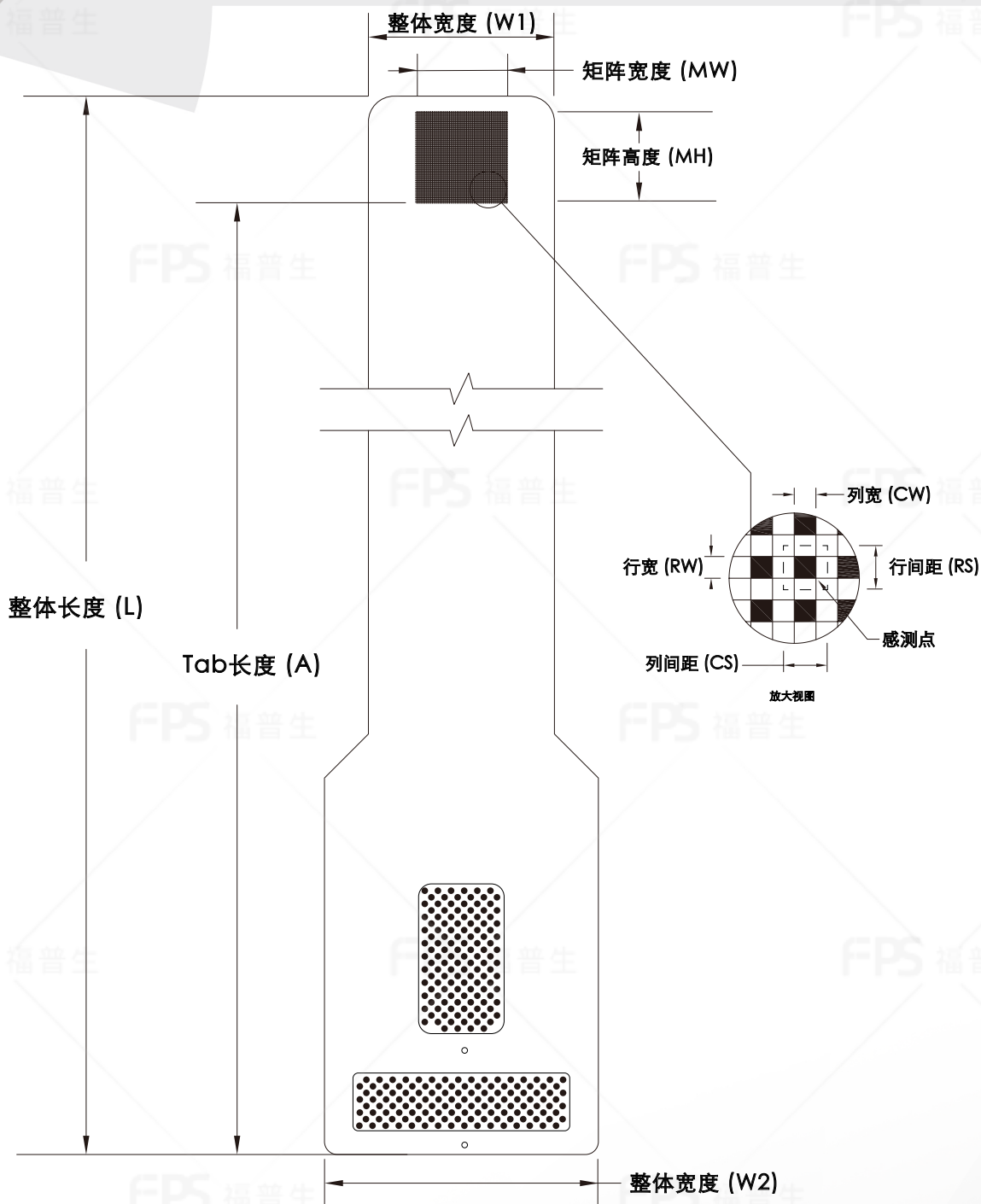
外形尺寸
