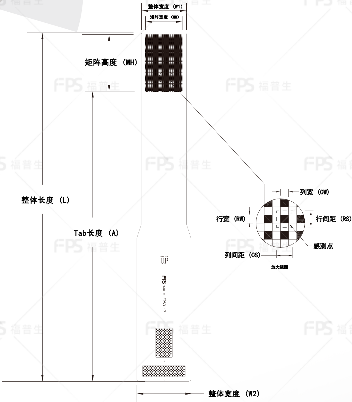
外形尺寸
