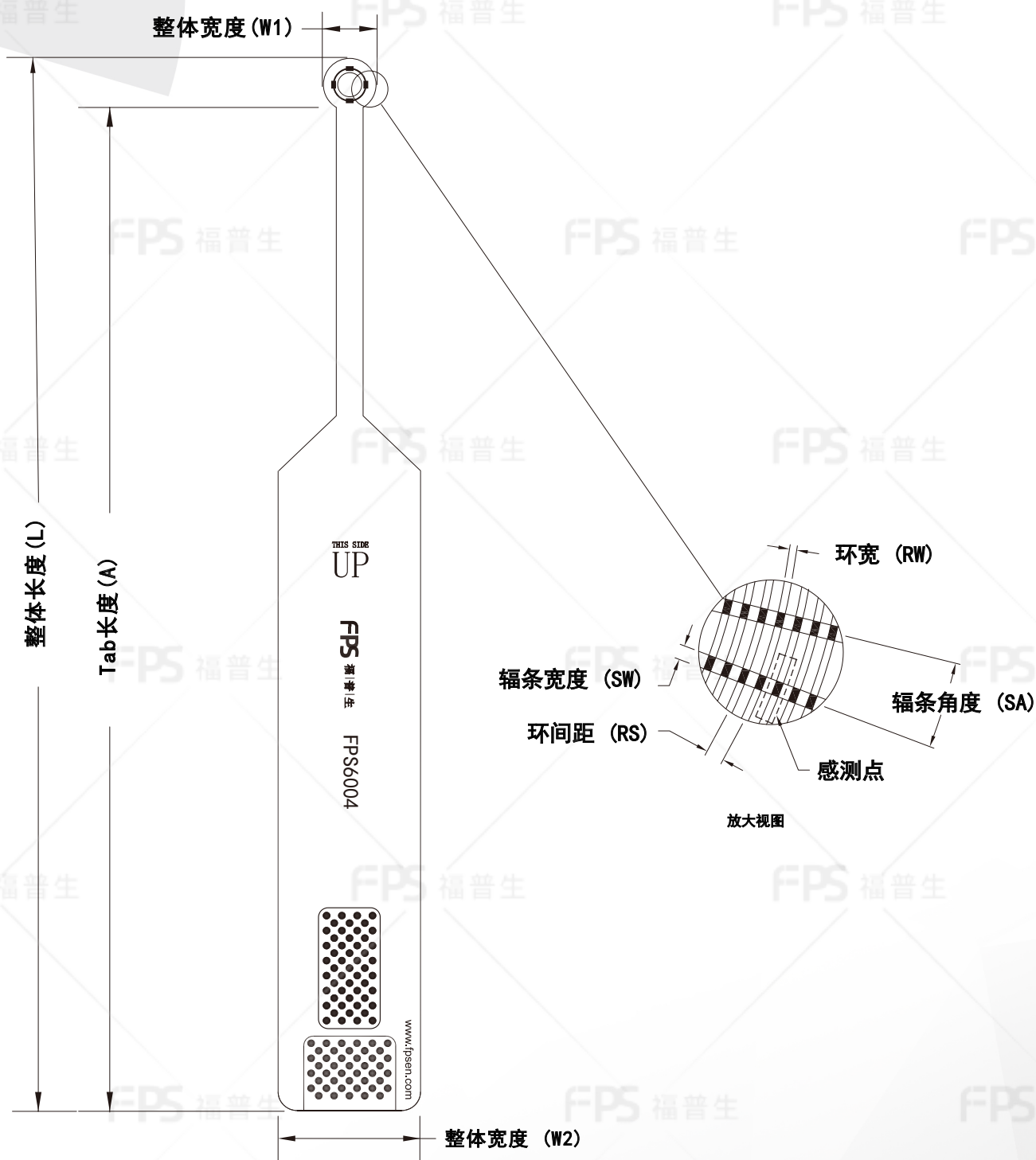
外形尺寸
