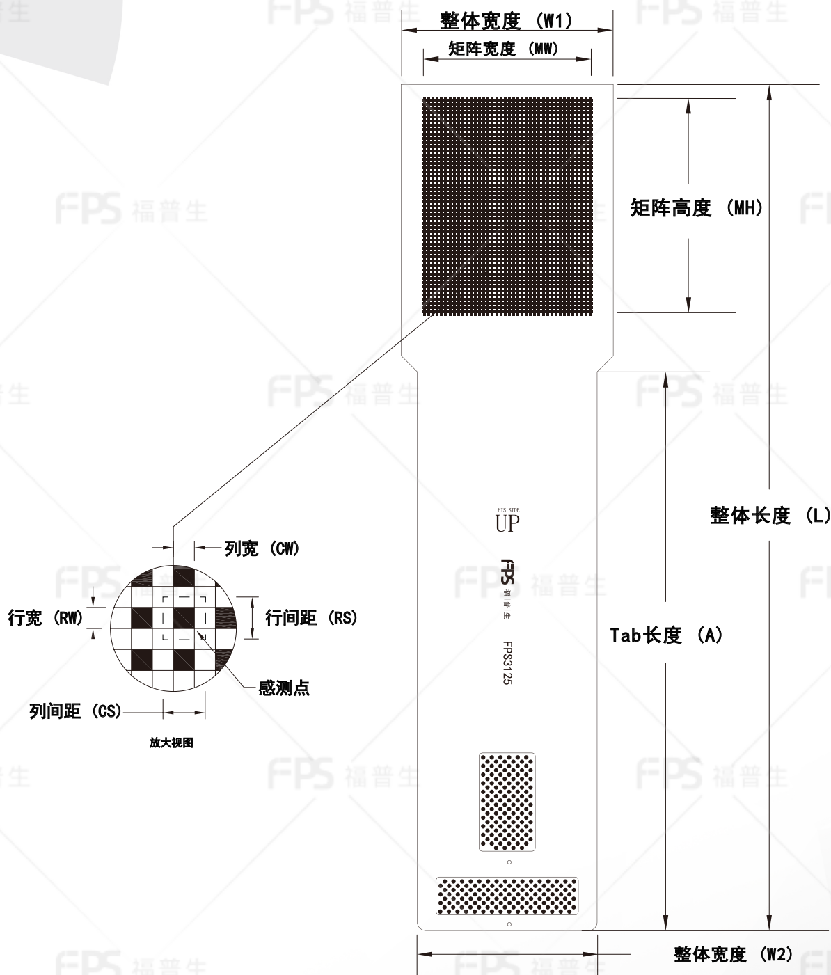
外形尺寸
