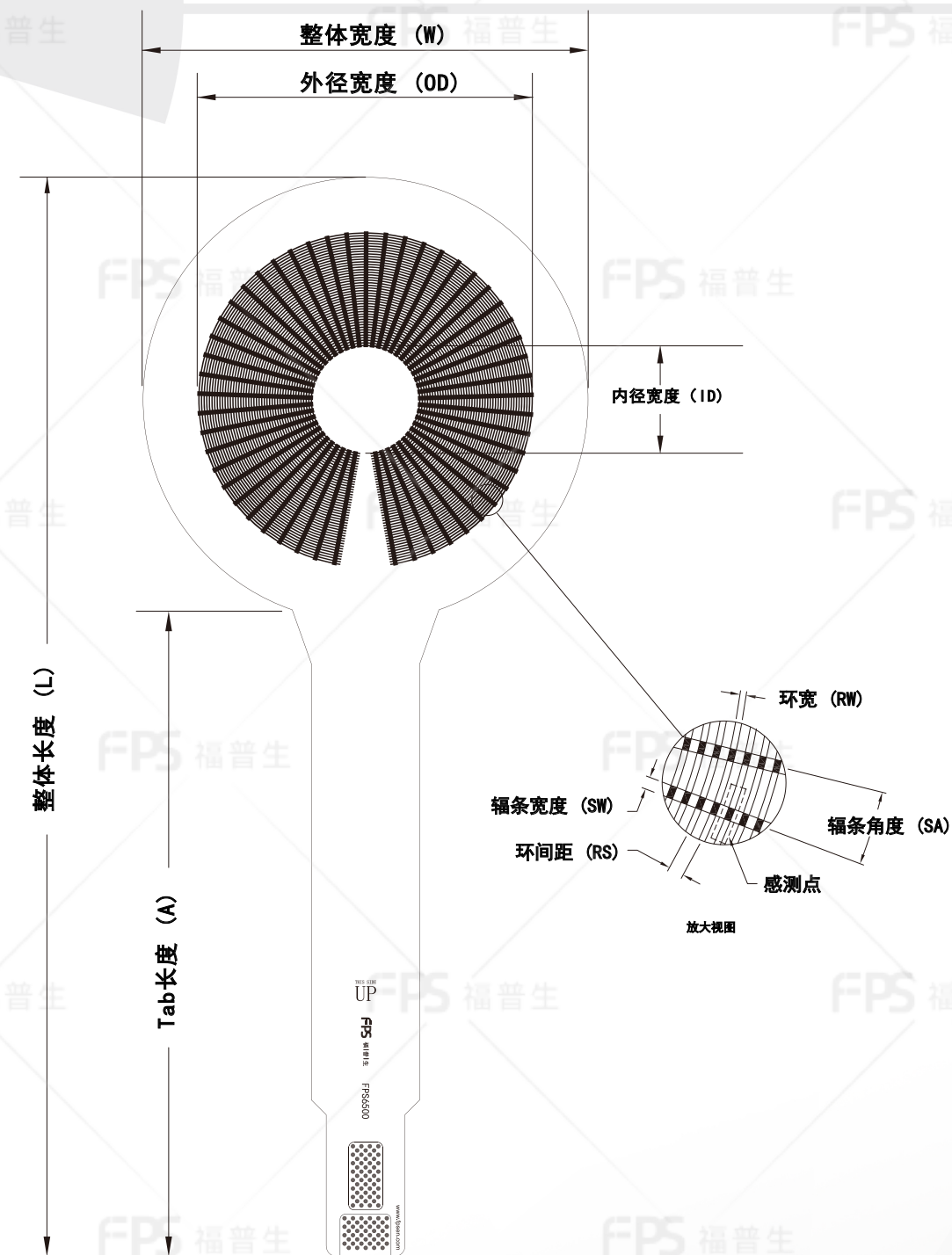
外形尺寸
