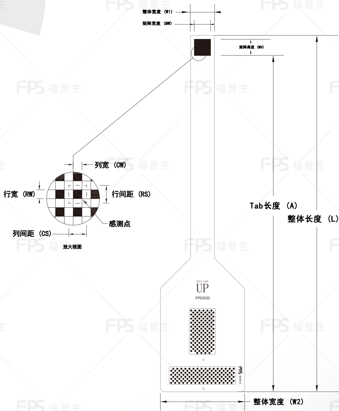
外形尺寸
