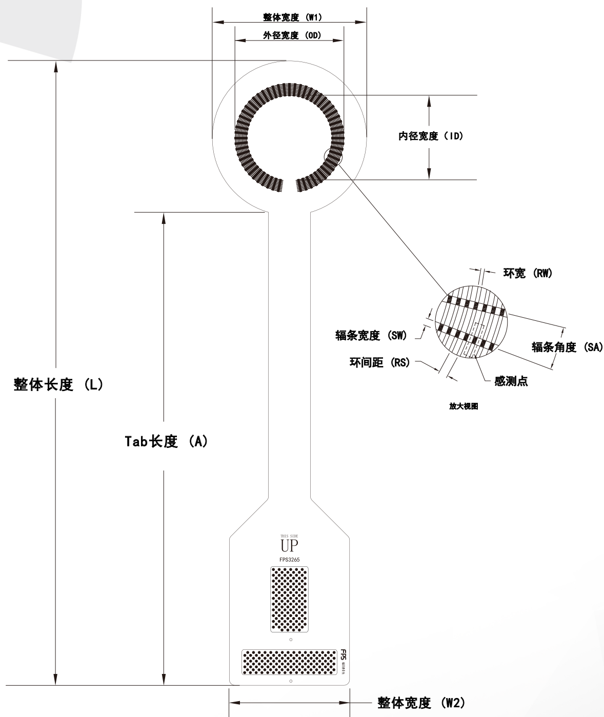
外形尺寸
