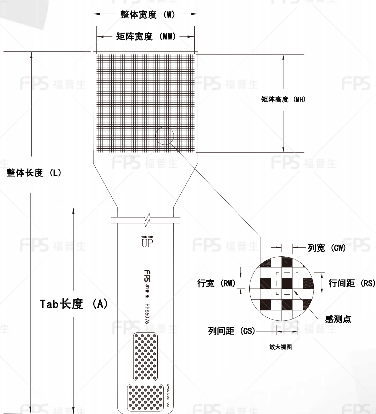
外形尺寸
