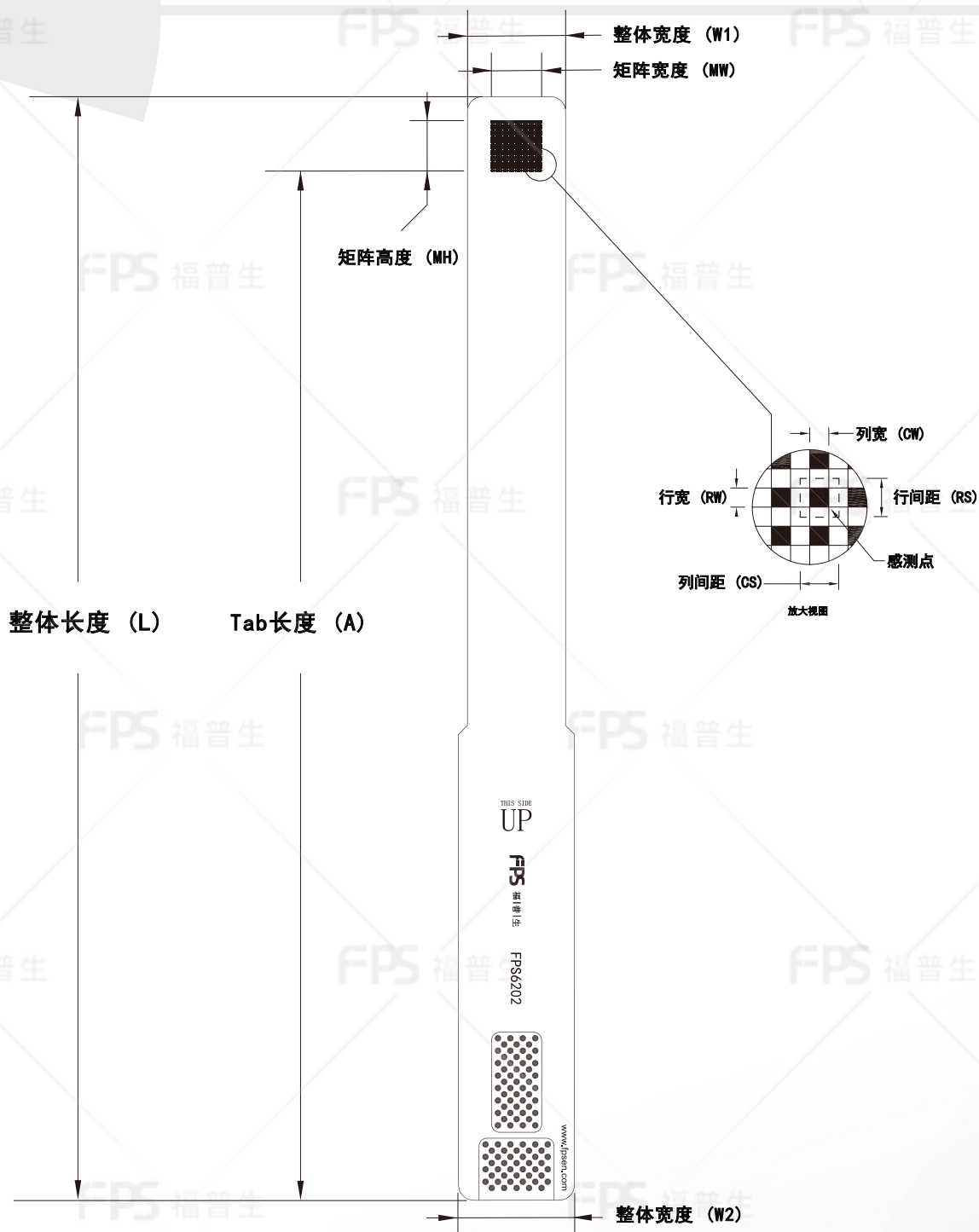
外形尺寸
