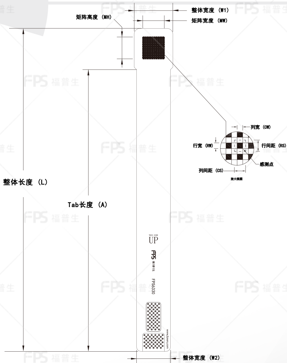
外形尺寸
