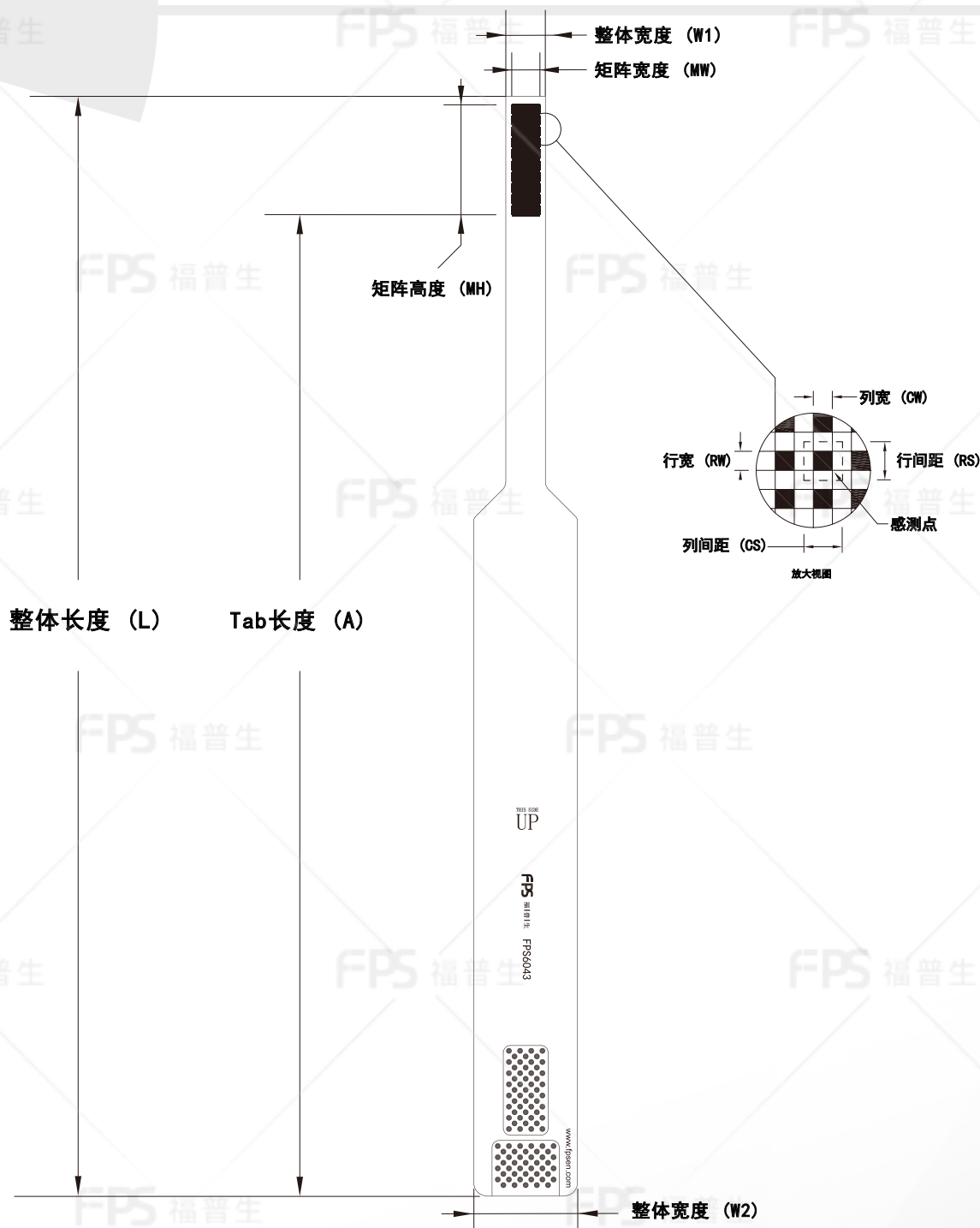
外形尺寸
