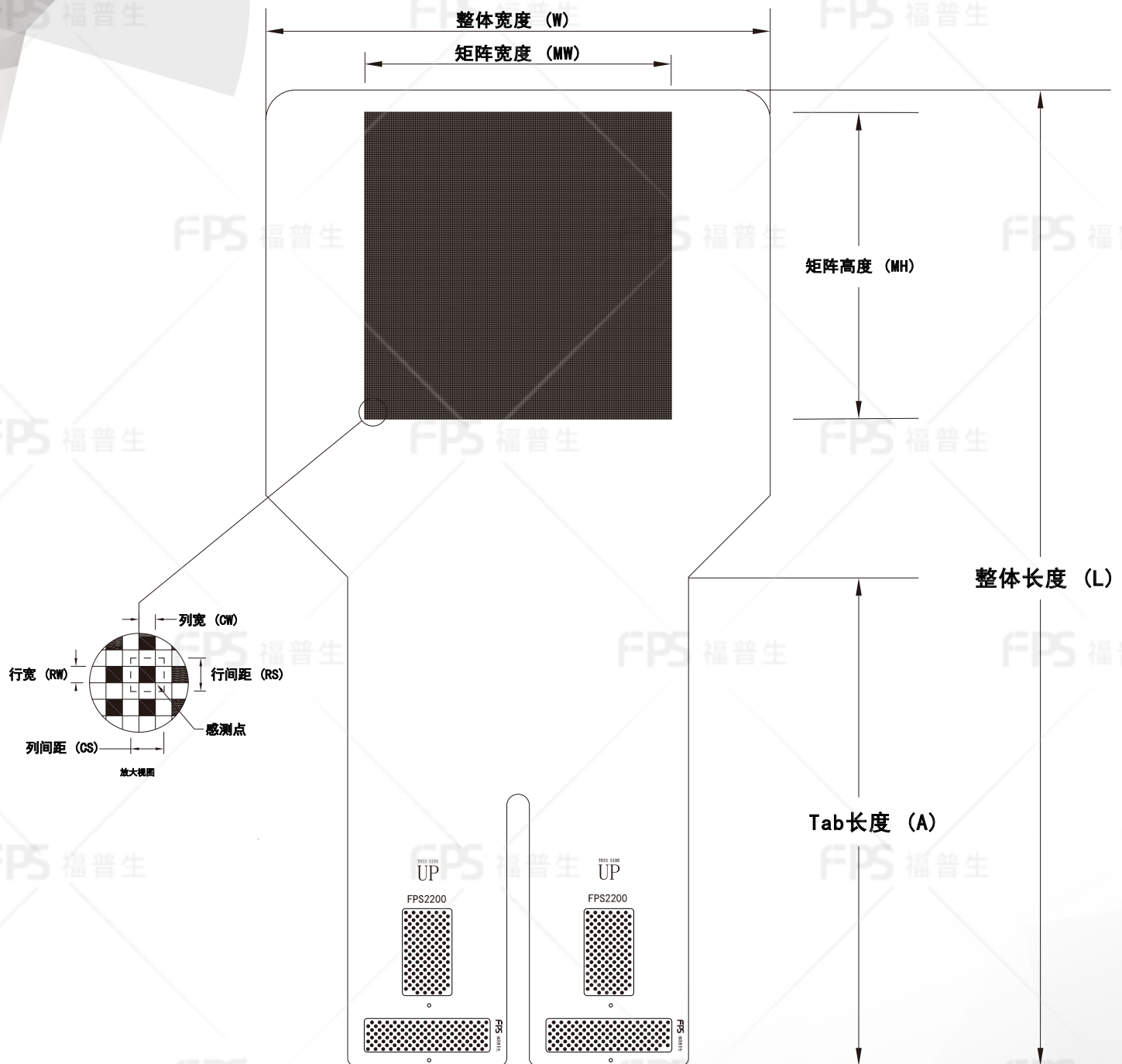
外形尺寸
