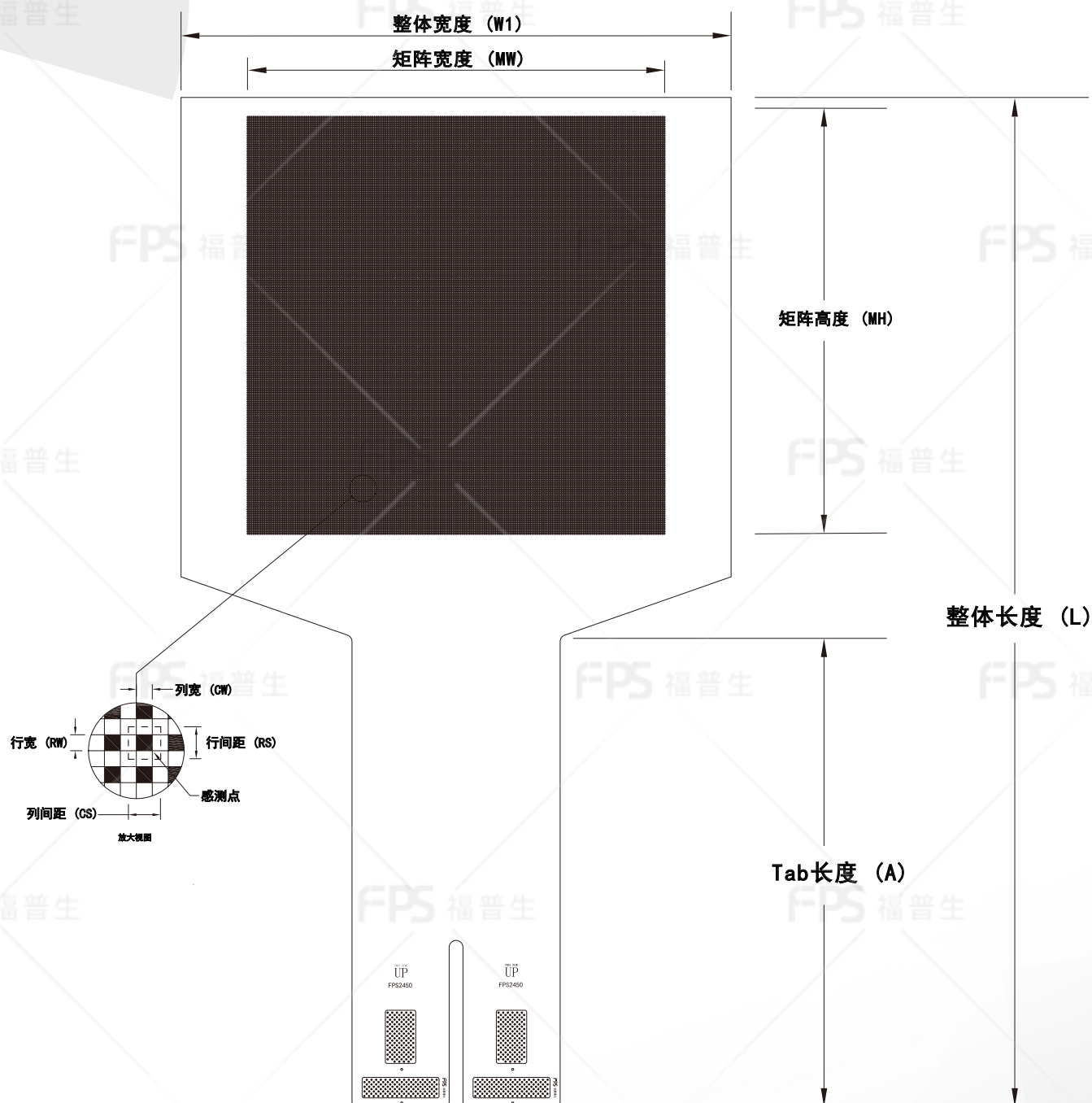
外形尺寸
